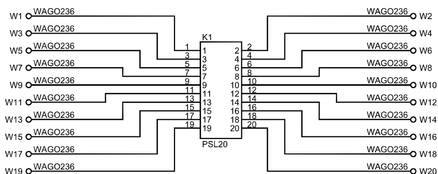
Obrázek 1: Schéma zapojení KA20
