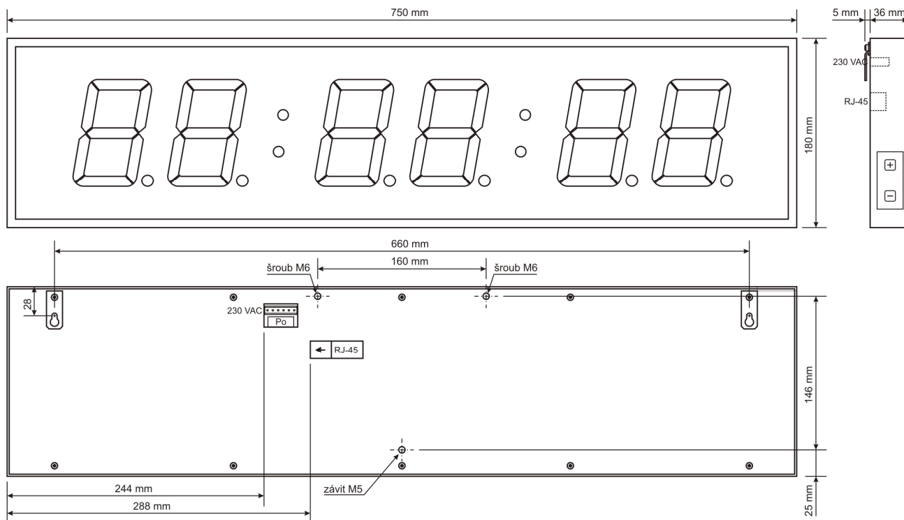
Obrázek 2: Rozměry DT100-6R-E (montáž na stěnu)
