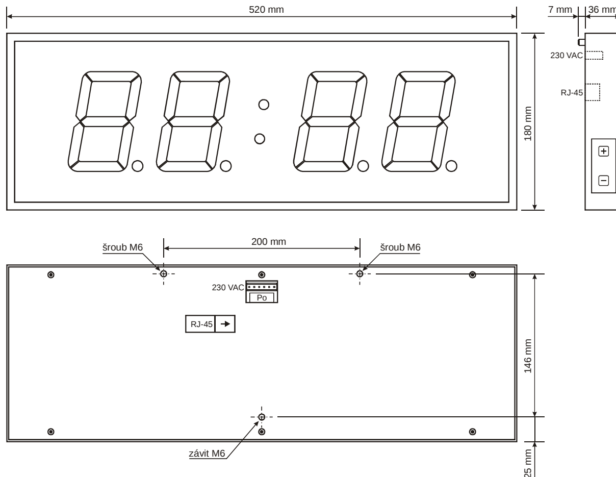
Obrázek 2: Rozměry DT100-4R-E (montáž na stěnu)
